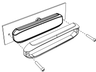
Skruvmontering med sarg
