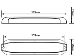
Måtten ovan är inklusive sarg. Mått för enbart varningsljus (BxHxD): 100x23x10mm
